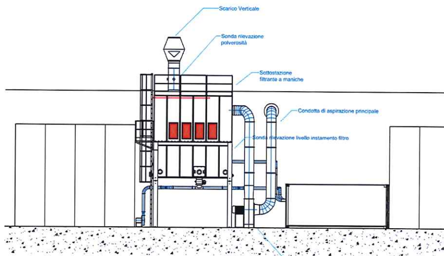
Fig. 1 – Componenti principali presenti negli impianto di aspirazione Mogentale 4.0 prodotti e venduti da Mogentale s.r.l .
