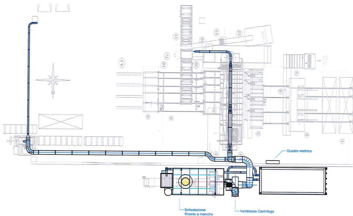
Fig. 2 – Esempio di impianto di aspirazione Mogentale 4.0 prodotto e venduto da Mogentale s.r.l. integrato all'interno di un'ambiente produttivo.
